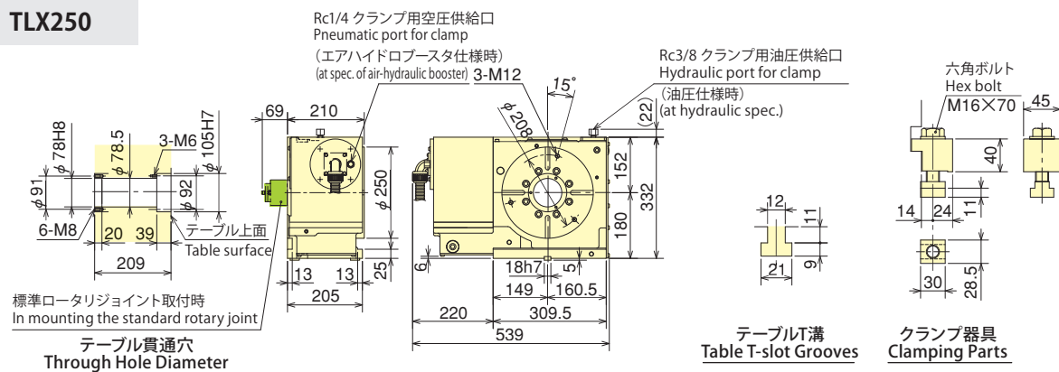
TRX320 (TLX)
