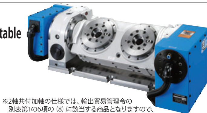
TW2180
