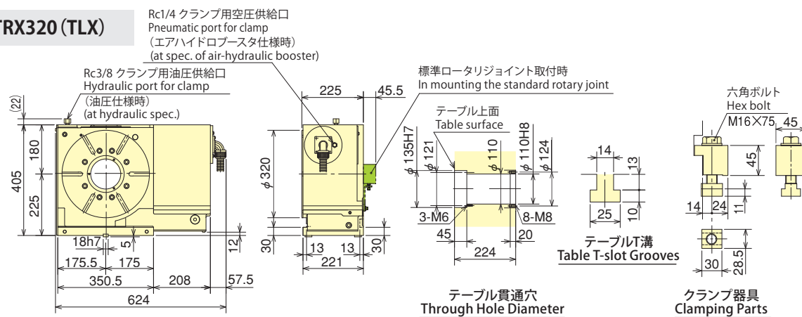
TR400 (TL)
