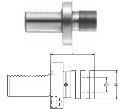
VDI Shank (VDI 3425/DIN 69880)
