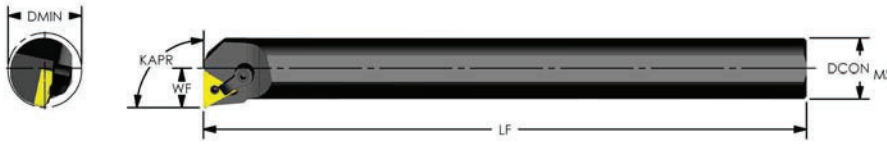
Negative Triangle (KAPR: 90°)
