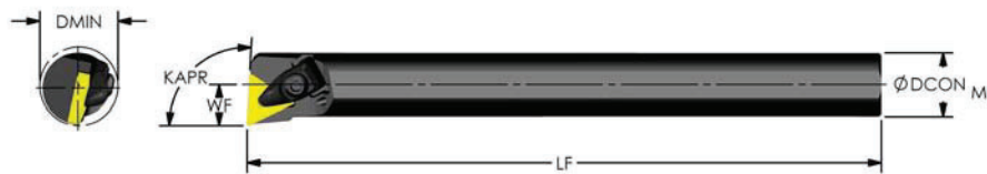
Negative Triangle (KAPR: 93°)
