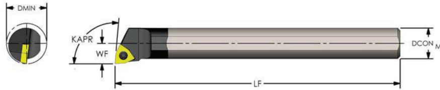
Positive Trigon (KAPR: 95°)
