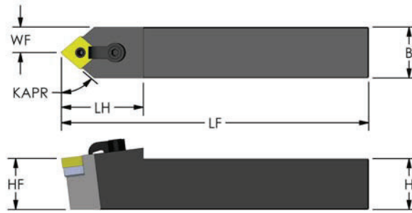
Negative 80° Diamond (KAPR: 50°)
