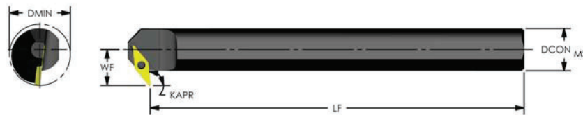
Positive 35° Diamond (KAPR: 95°) Back Facing
