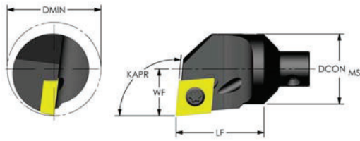
Positive 80° Diamond (KAPR: 95°)
