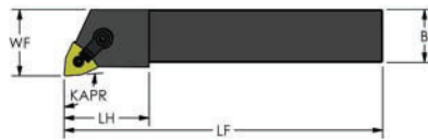
Negative Trigon (KAPR: 95°)
