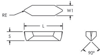
V-Bottom
